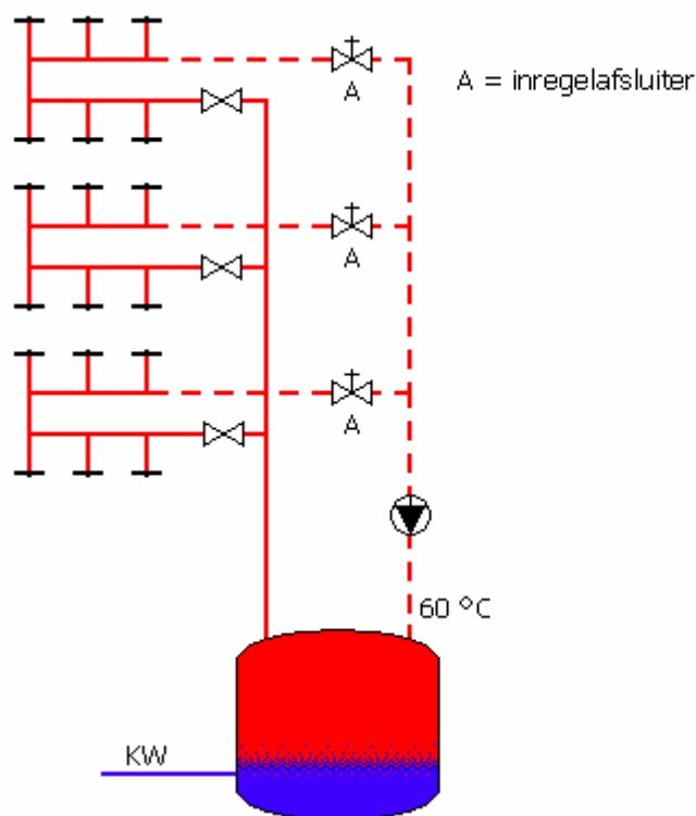
Figuur 1: Principeschema van een circulatiesysteem met deelringen
