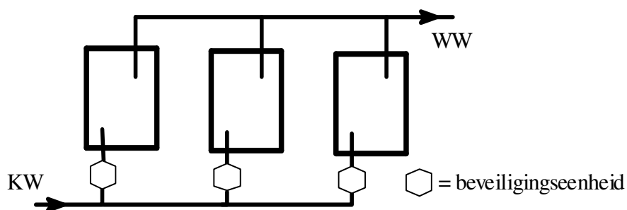
Figuur 1A: Principeschets Parallelschakeling
