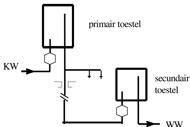
Figuur 1D: Principeschema's in serie geplaatst secundair warmtapwatertoestel
