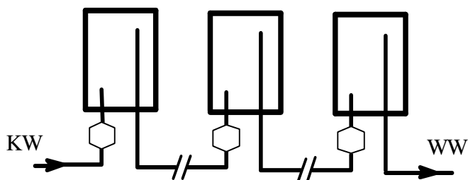
Figuur 1B: Principeschets Serieschakeling
