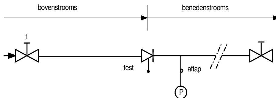
Figuur 1 Controleopstelling standaardmethode
