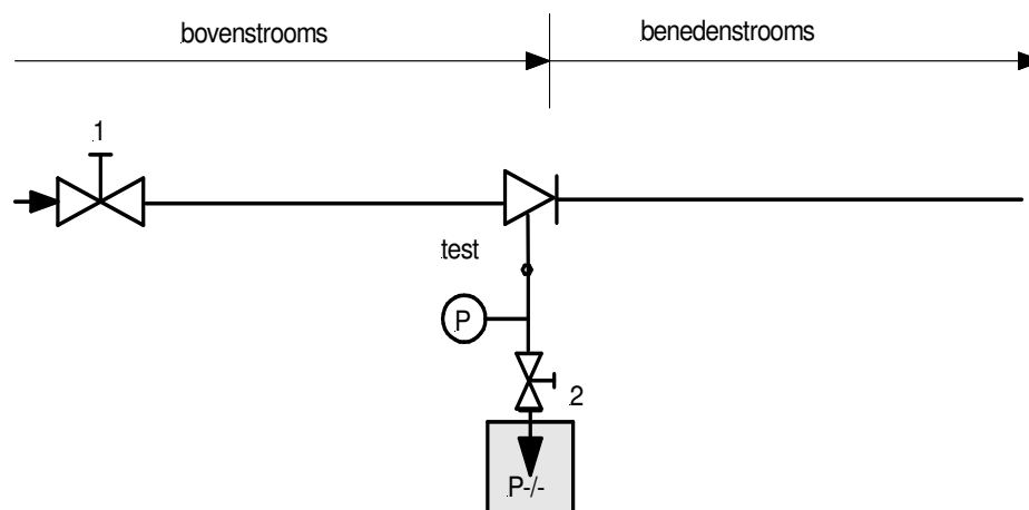
Figuur 2 Controleopstelling vacuümmethode
