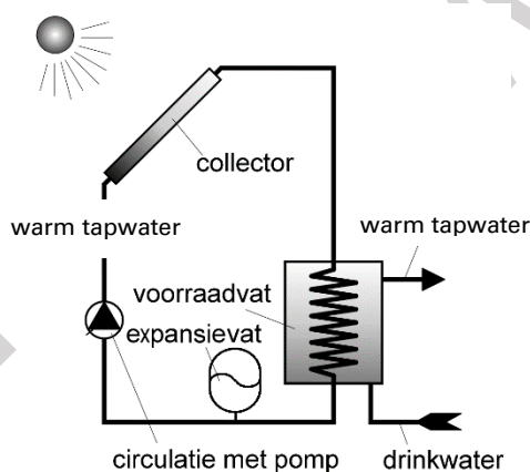
Figuur 1: Prinscheschets van circulatie met pomp in een geheel met vloeistof gevuld systeem
