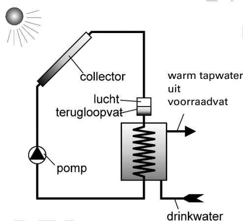
Figuur 2A: Principeschema terugloopstelsel met warm tapwater in voorraad
