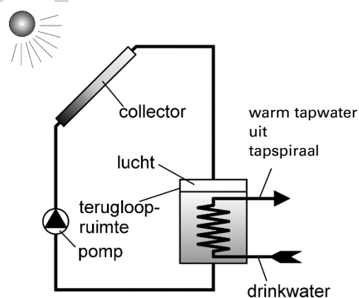
Figuur 2B: Principeschema terugloopstelsel met primair medium in voorraad
