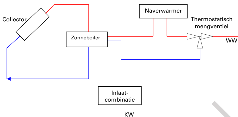
Figuur 5B Zonne-energiesysteem met thermostatisch mengventiel na de naverwarmer geplaatst
