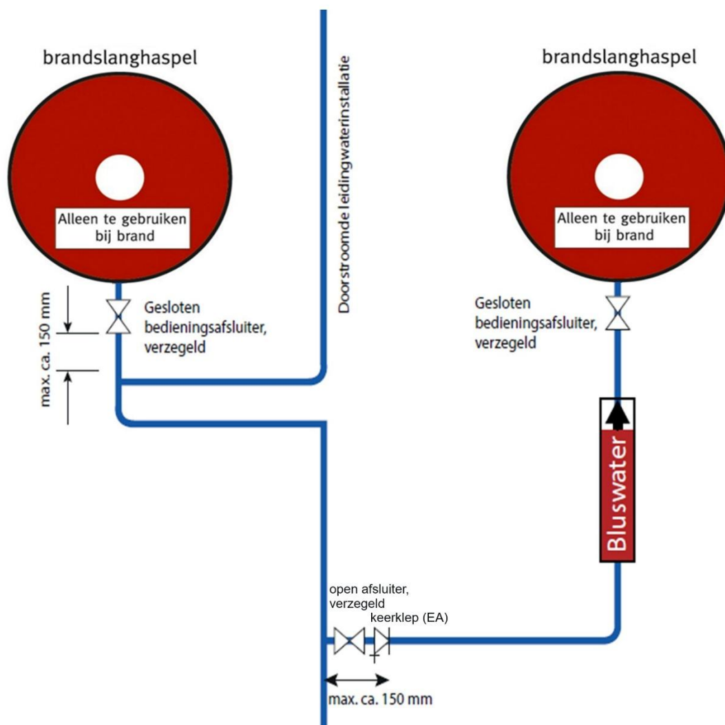
Figuur 2 Principeschets geen separate bluswaterleiding
