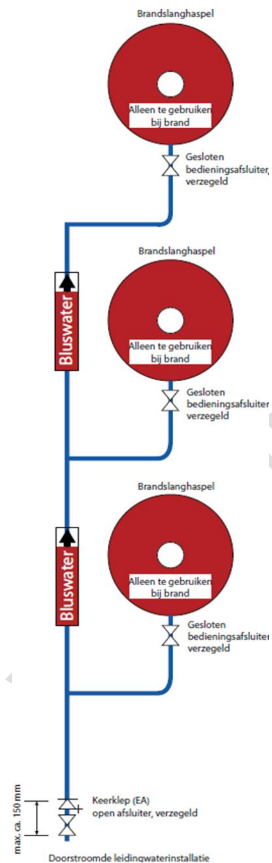
Figuur 1 Principeschets separate bluswaterleiding
