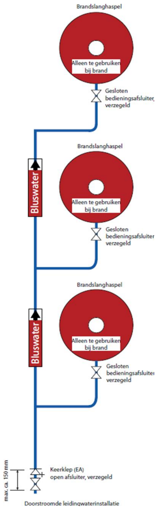
Figuur 1 Principeschets separate bluswaterleiding
