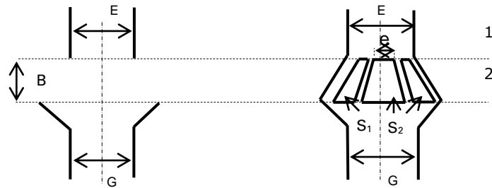
Figuur 1: Uitvoering aansluiting op gebouwrilering
