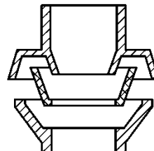
Figuur 12 Ontwerpprincipe terugstroombeveiliging DC
