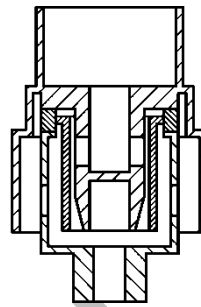
Figuur 11 Ontwerpprincipe terugstroombeveiliging DB
