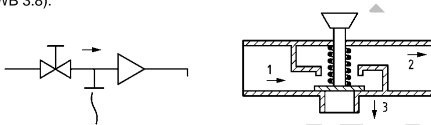
Figuur 9 Ontwerpprincipe terugstroombeveiliging HC
