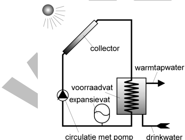
Figuur 1: Principeschets van circulatie met pomp in een geheel met vloeistof gevuld systeem
