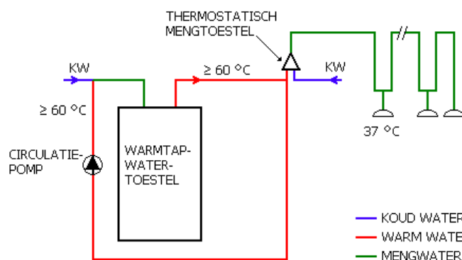
Figuur 5: Prinschesets van een mengwaterinstallatie
