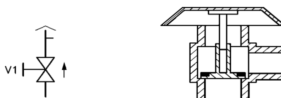
Figuur 10 Ontwerpprincipe terugstroombeveiliging DA
