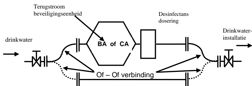
Figuur 1: Of-Of verbinding tijdens desinfecteren of reinigen
