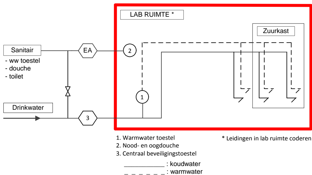
Figuur 1: Voorbeeld van een laboratorium met een eigen warmtapwater-voorziening voor het proceswater in de laboratoriumruimte
