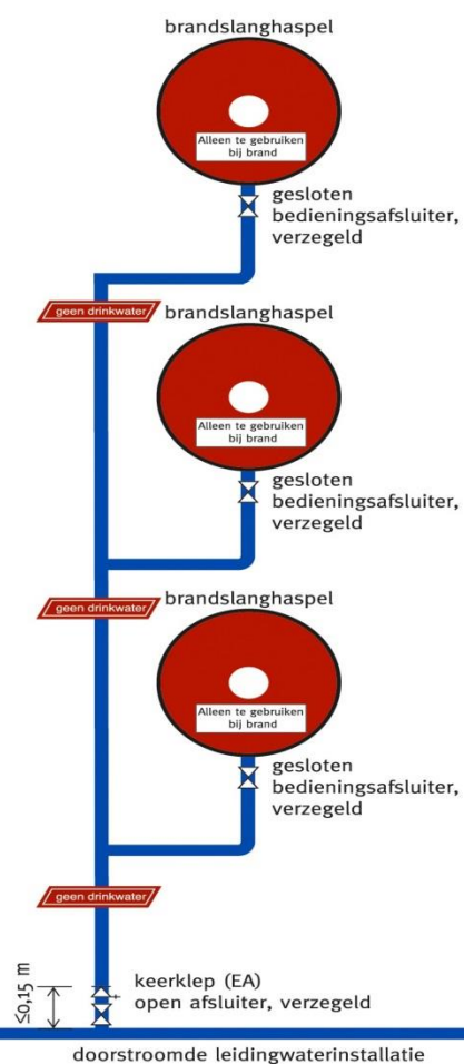
Figuur 1 Principeschets separate bluswaterleiding
