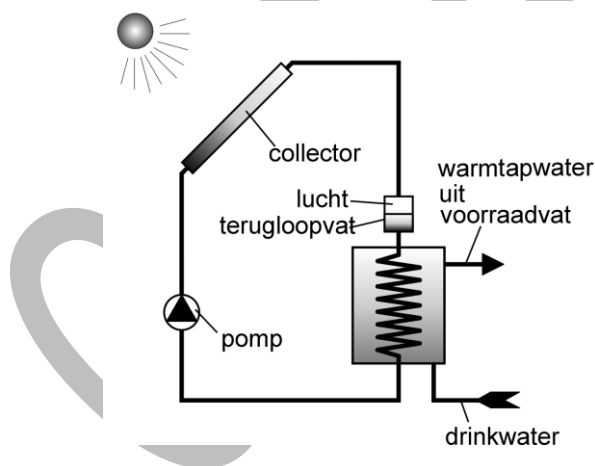
Figuur 2 A: Principeschets terugloopsysteem met warmtapwater in voorraad
