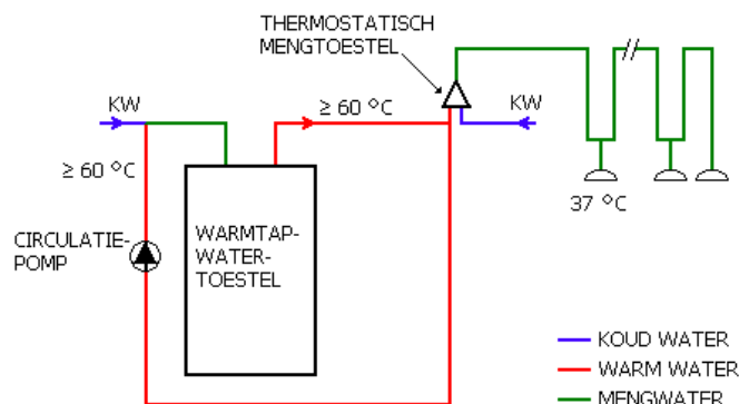
Figuur 5: Prinschesets van een mengwaterinstallatie
