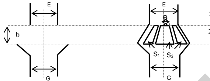
Figuur 1: Uitvoering aansluiting op gebouwriolering
