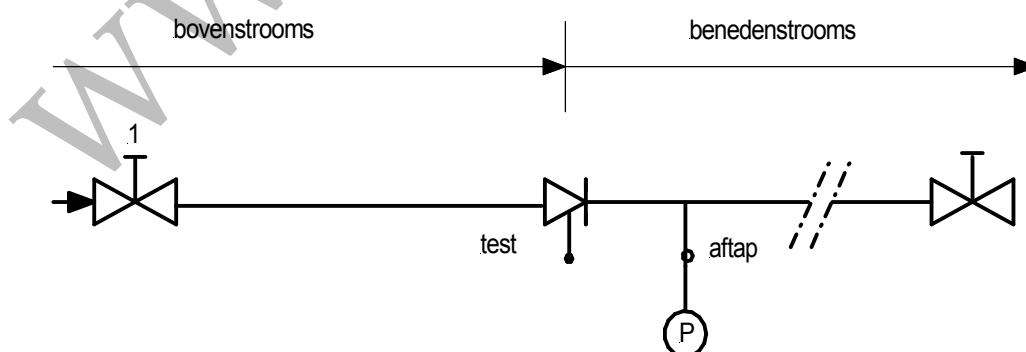
Figuur 1 Controleopstelling standaardmethode
