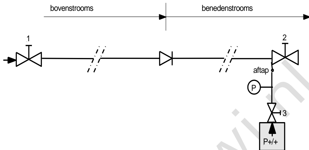
Figuur 3 Controleopstelling overdrukmethodede
